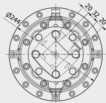
B-B
