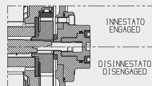
DETTAGLIO DISINNESTO DISENGAGEMENT DETAIL
