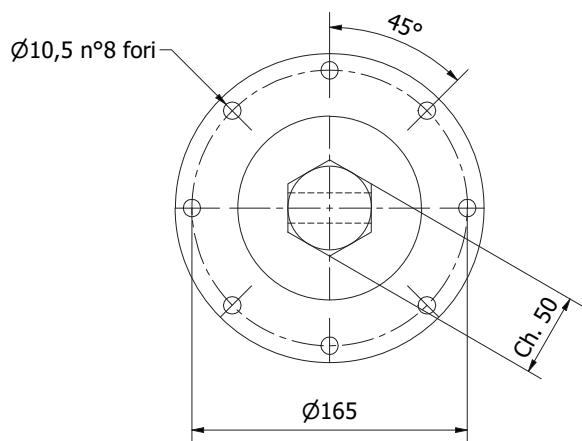
Vista A
