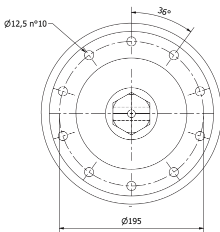
Vista A
