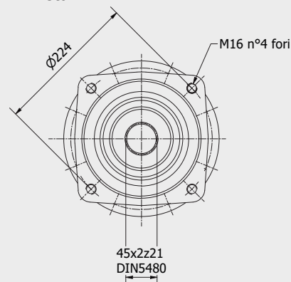
Vista A
