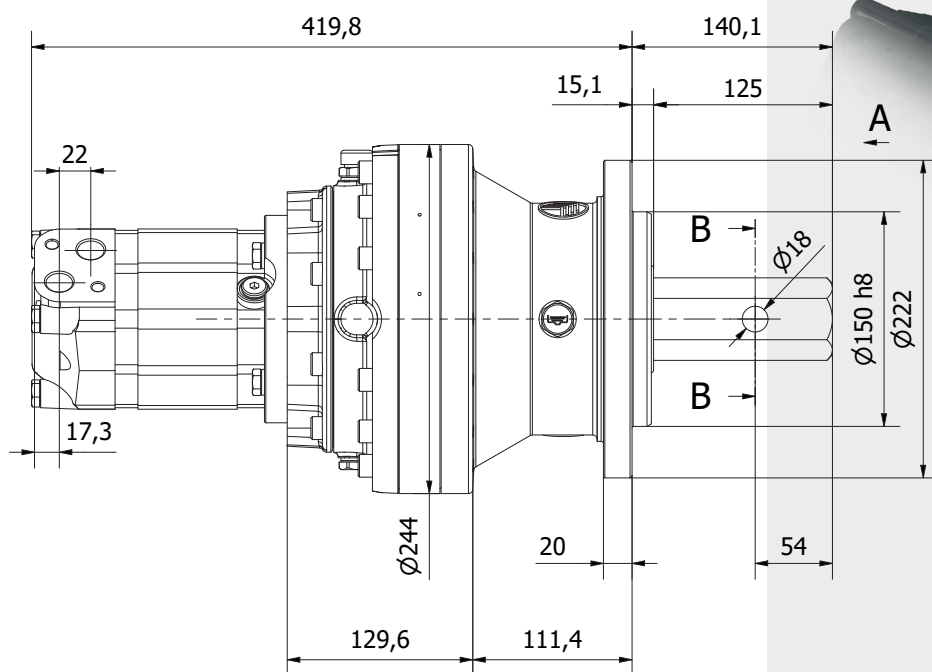
Vista A
