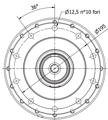
Vista B
