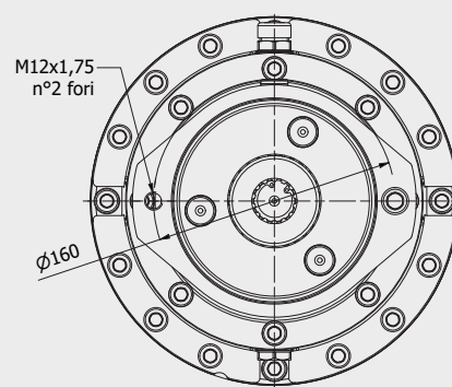
Vista A
