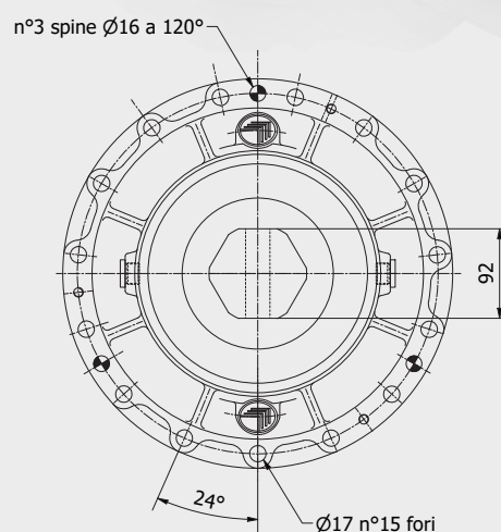
Vista B
